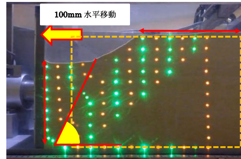
図-2 計測手順
