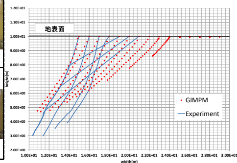
図-7 数値解析と実験結果の地表面の軌跡比較図
