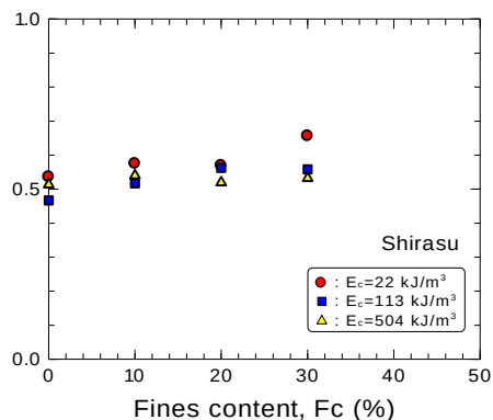
図-3. 実験定数 n と細粒分含有率の関係
