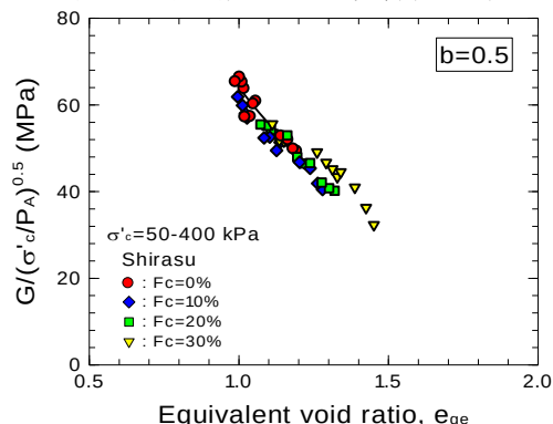
図-4. 平均有効主応力で正規化したせん断弾性係数と等価骨格間隙比の関係
