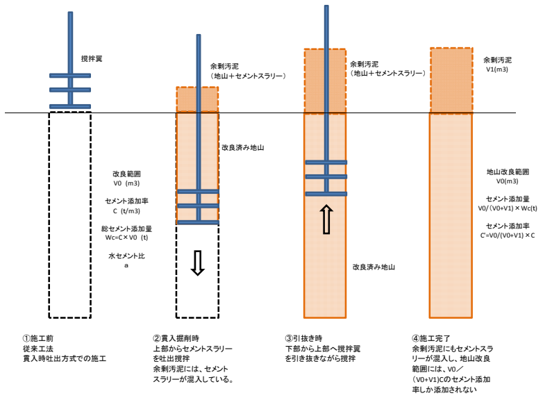
図-4 従来工法の施工イメージ
