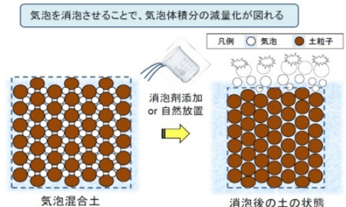
図-3 消泡による残土量低減の模式図
