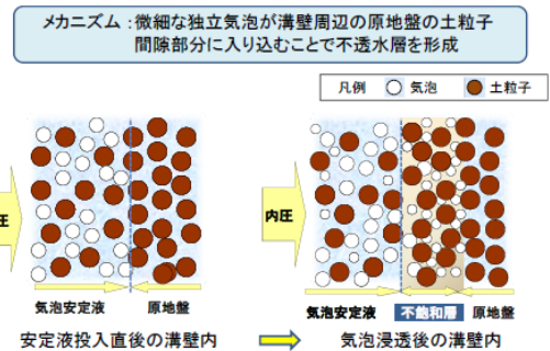
図-1 溝壁安定性の模式図
