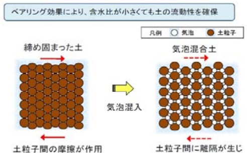
図-2 気泡によるベアリング効果の模式図
