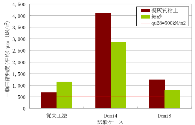
図-1 一軸圧縮強度試験結果
