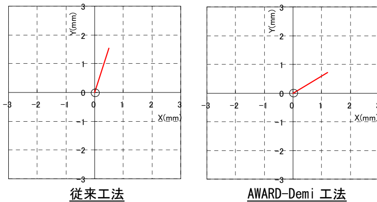
図-6 地中変位計測結果（平面図）
