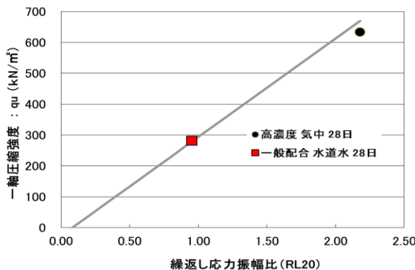
図 3.3 q_u \sim R_{L20} の関係
