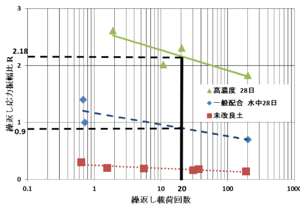
図 3.2 繰返し非排水三軸試験結果
